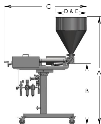
SP-160 con puerto delantero, boquilla de 2" y tolva con agitación
